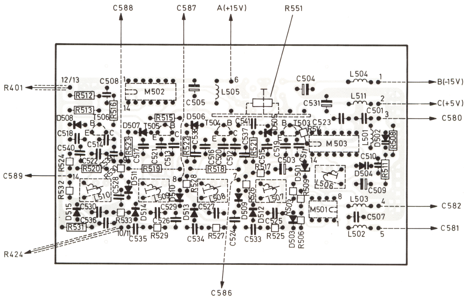
Oszillatorplatine AS 30 Unbestückte Seite – 493.041/A
